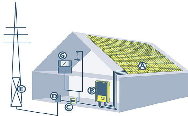
A ΦΩΤΟΒΟΛΤΑΙΚΑ ΠΛΑΙΣΙΑ B ΑΝΤΙΣΤΡΟΦΕΑΣ ΙΣΧΥΟΣ C ΜΕΤΡΗΤΗΣ ΕΝΕΡΓΕΙΑΣ D ΣΗΜΕΙΟ ΣΥΝΔΕΣΗΣ ΜΕ ΤΟ ΔΙΚΤΥΟ E ΔΗΜΟΣΙΟ ΔΙΚΤΥΟ G ΦΟΡΤΙΑ
